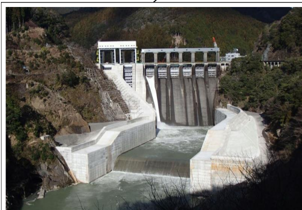
長安ダム改造事業 新設洪水吐ゲート 令和元年度より運用開始
