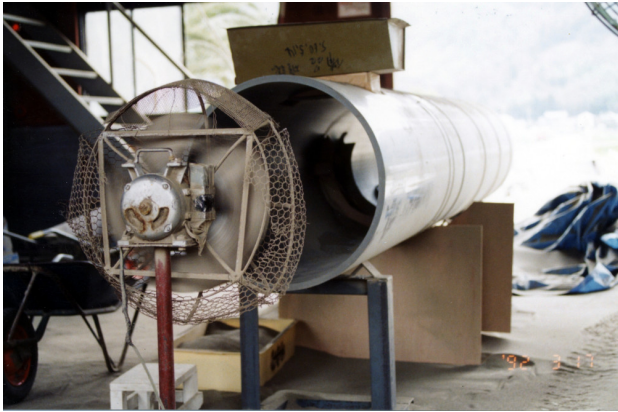
写真2-6-7 風選処理
