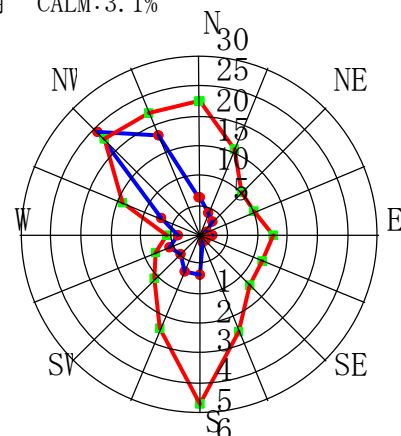
3月 CALM:3.0%
