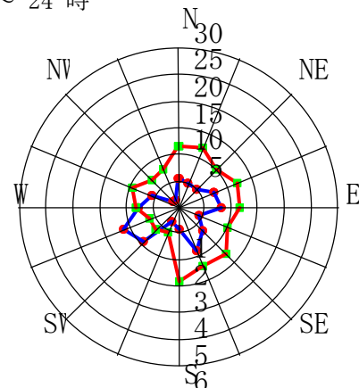
6月 CALM:7.0%
