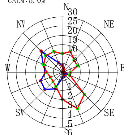
11月 CALM:3.6%
