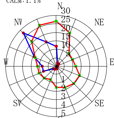
1月 CALM:0.5%
