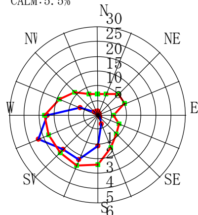
12月 CALM:1.6%
