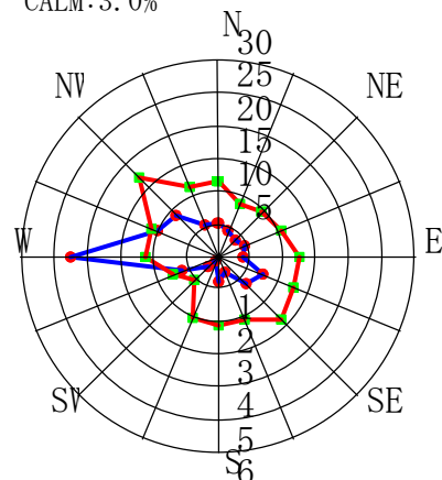
9月 CALM:3.8%
