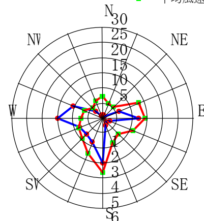
7月 CALM:4.4%
