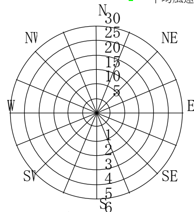
7月 CALM:0.0%
