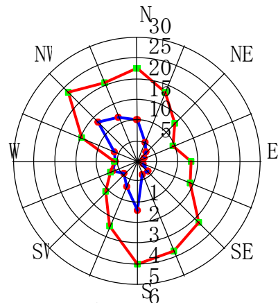
4月 CALM:4.5%
