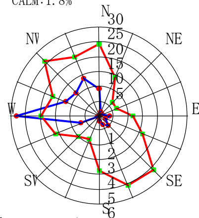
10月 CALM:0.5%
