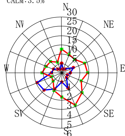
8月 CALM:5.5%
