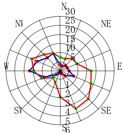
4月 CALM:1.8%
