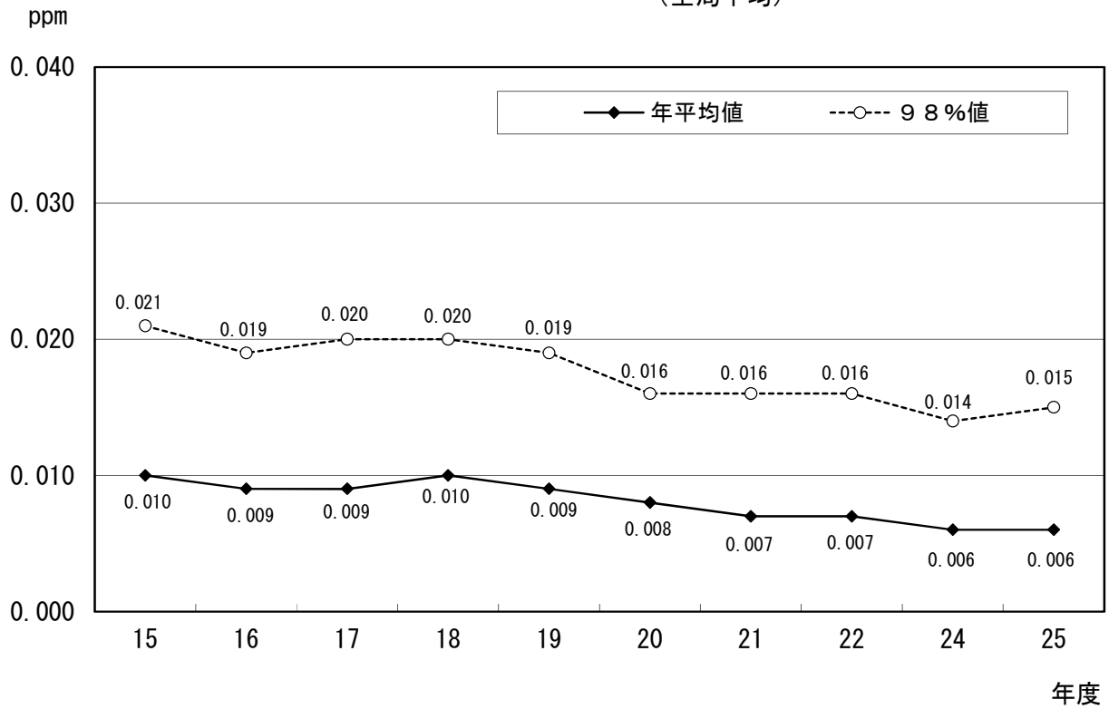
図Ⅱ-2-1 二酸化窒素の経年変化 (全局平均)
