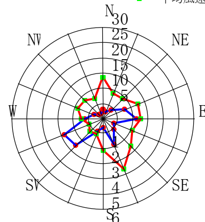
7月 CALM:7.3%
