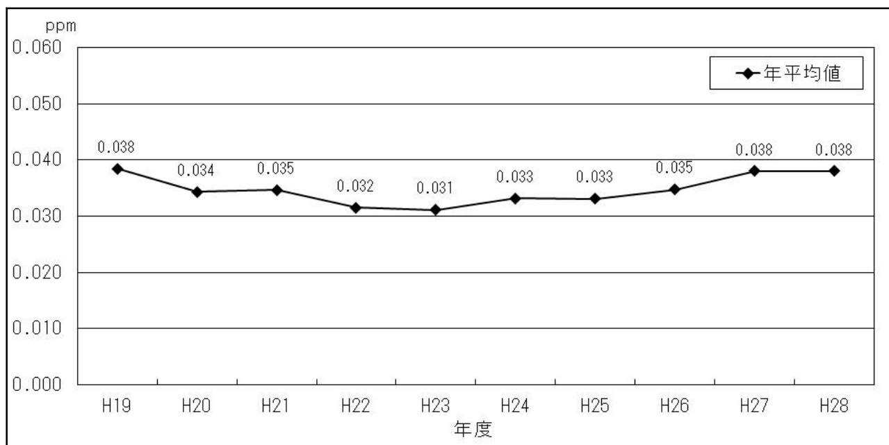
図Ⅱ－3－1 光化学オキシダント(Ox)の経年変化(全局平均)
