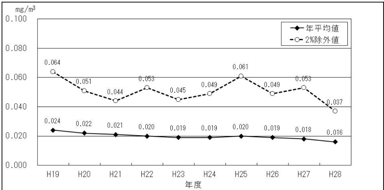
図Ⅱ－４－１ 浮遊粒子状物質の経年変化(全局平均)
