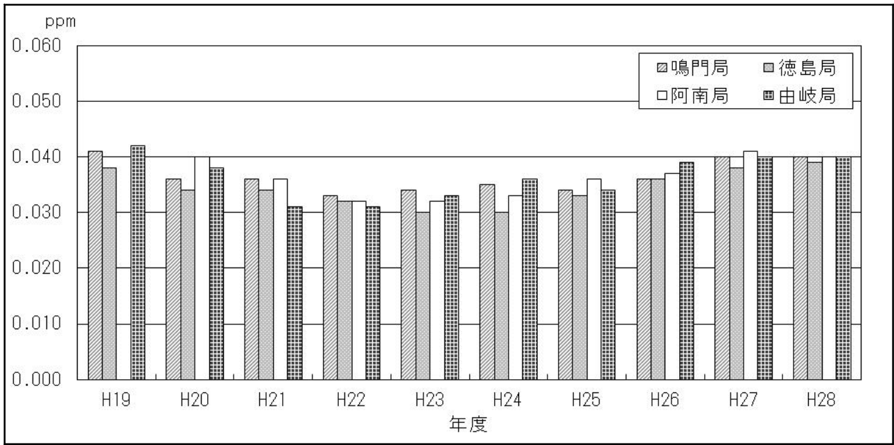
図Ⅱ－３－２ 光化学オキシダント年平均値の経年変化
