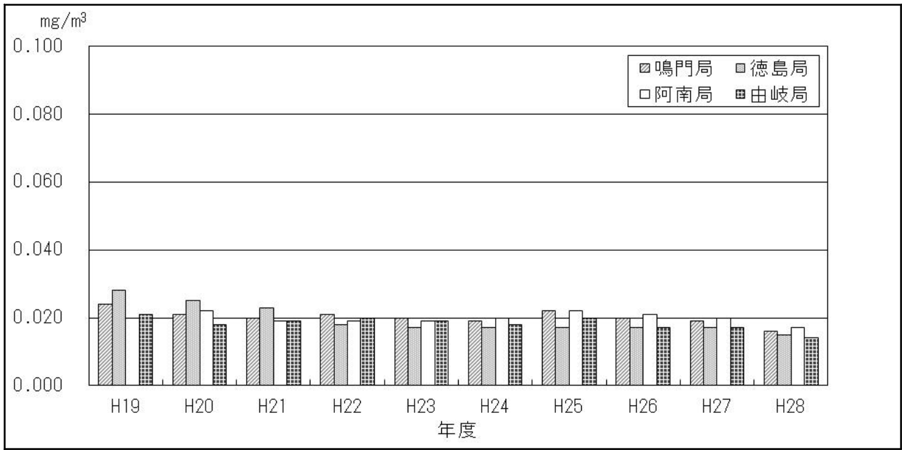
図Ⅱ－４－２ 浮遊粒子状物質年平均値の経年変化
