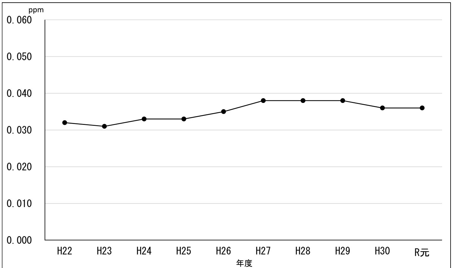
図Ⅱ-3-1 光化学オキシダント(Ox)の昼間の1時間値の全局年平均値の経年変化
