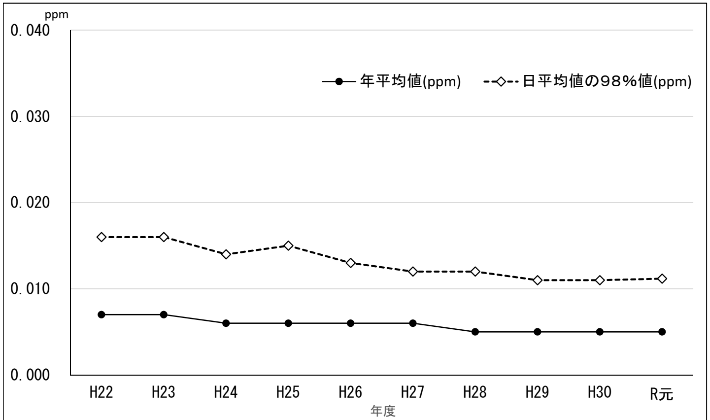
図 II - 2 - 1 二酸化窒素の経年変化(全局平均)
