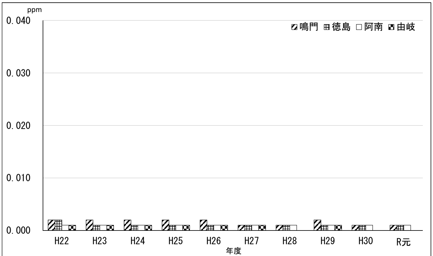
図 II - 1 - 2 二酸化硫黄(SO 2 )年平均値の経年変化
