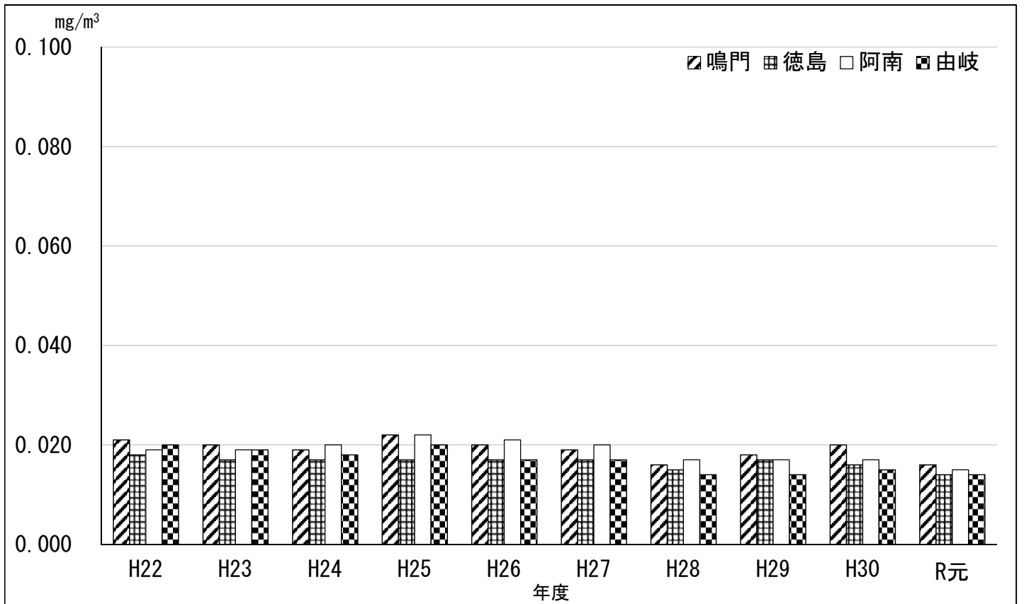
図 II - 4 - 2 浮遊粒子状物質年平均値の経年変化
