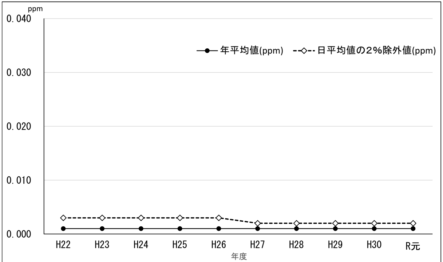
図 II - 1 - 1 二酸化硫黄(SO 2 )の経年変化(全局平均)
