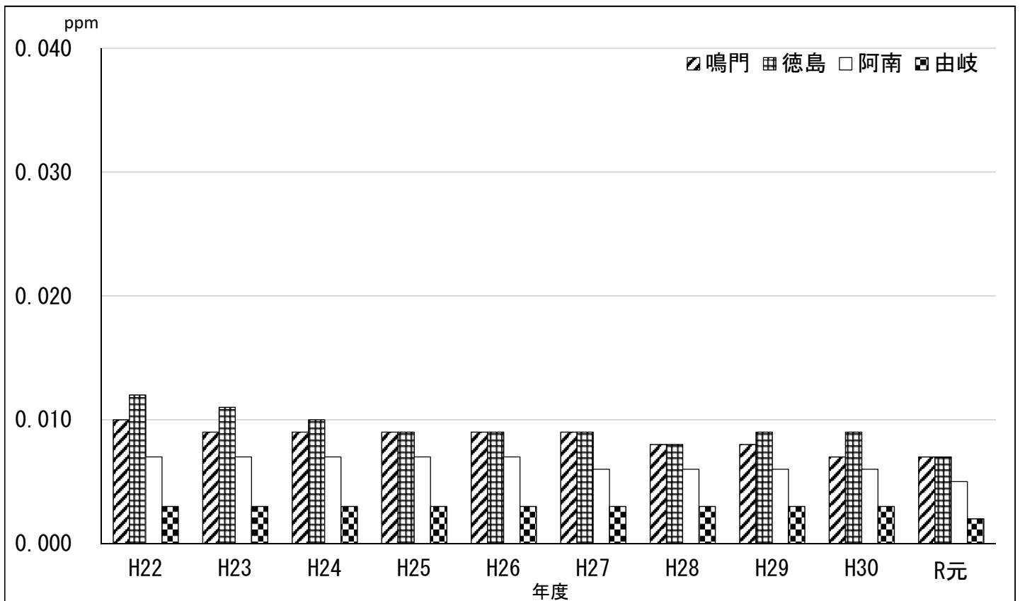
図 II - 2 - 2 二酸化窒素年平均値の経年変化
