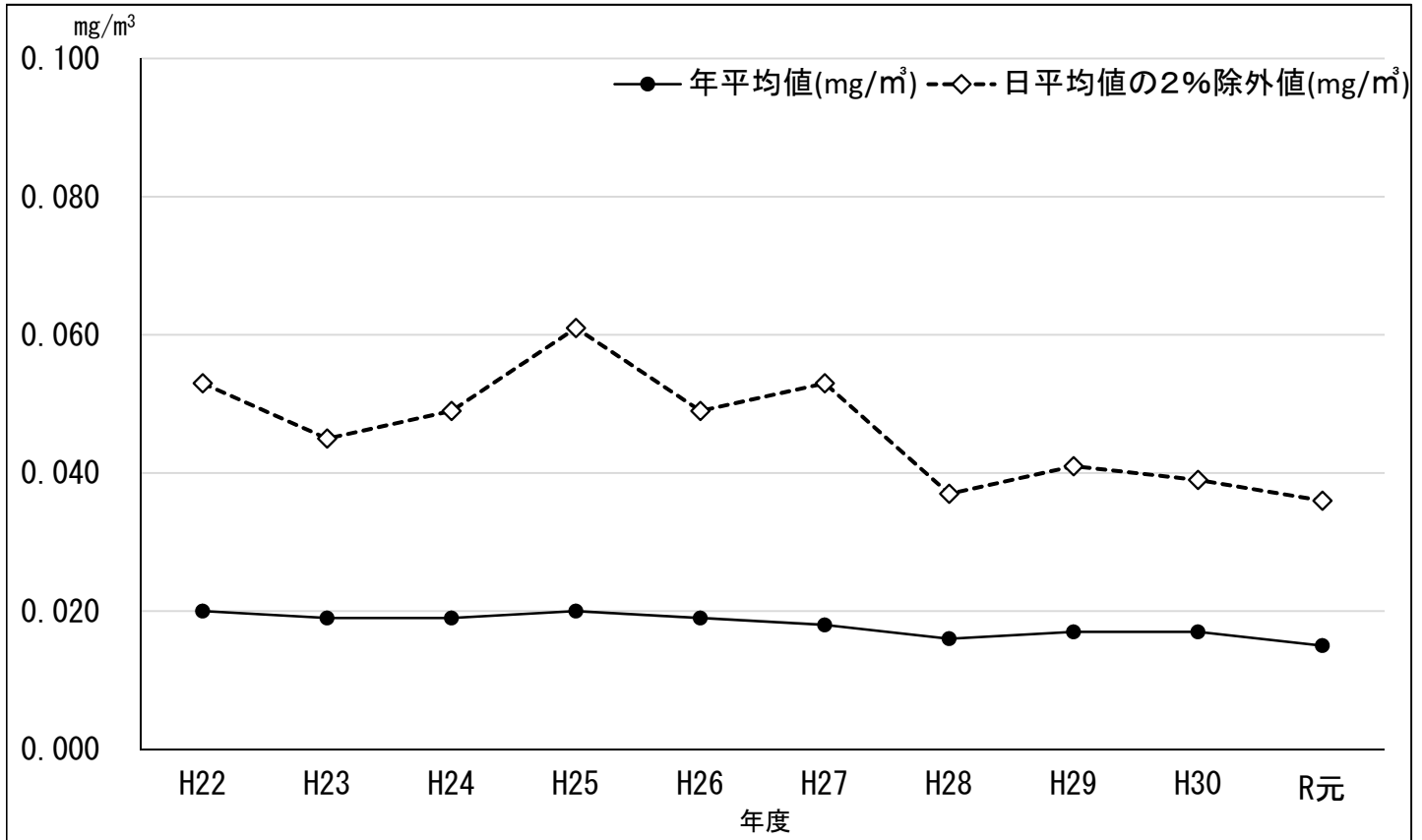
図 II - 4 - 1 浮遊粒子状物質の経年変化(全局平均)
