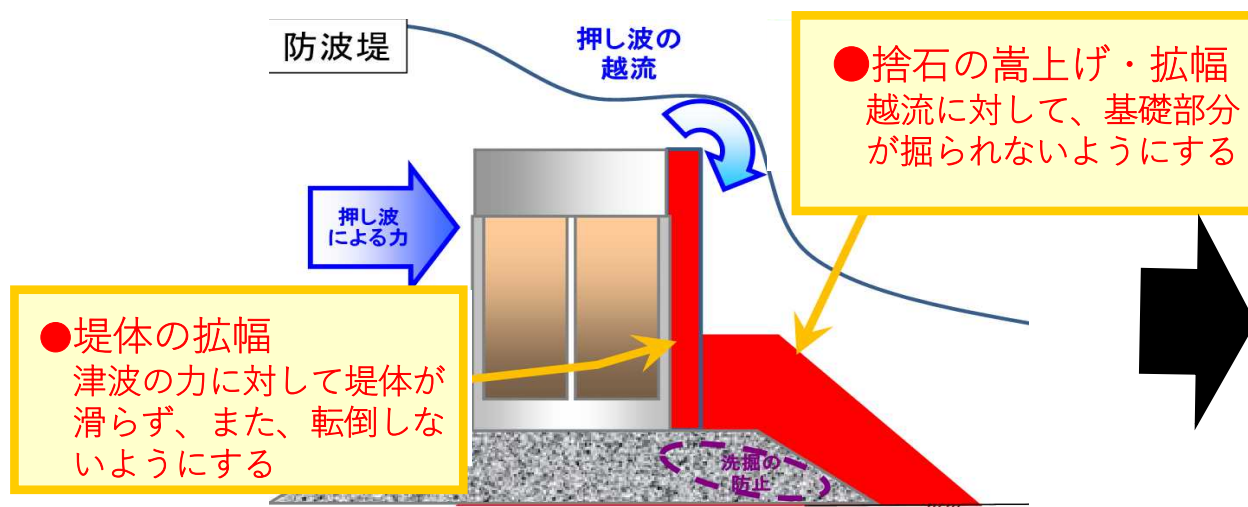
【防波堤の粘り強い化イメージ】
