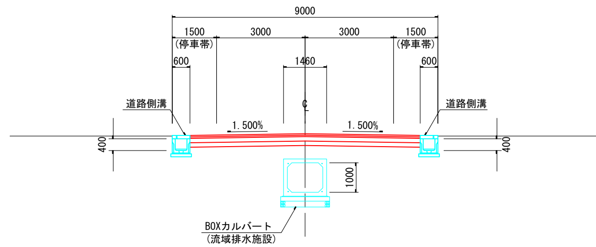
区画道路 3, 4
