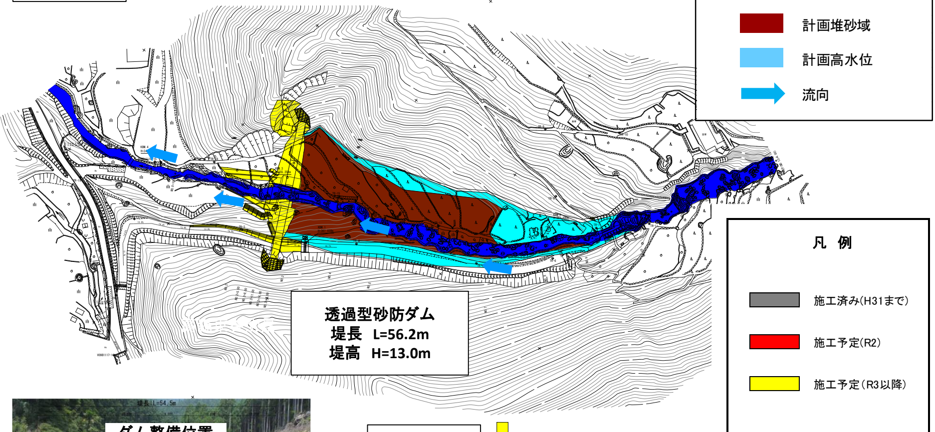
一般図
