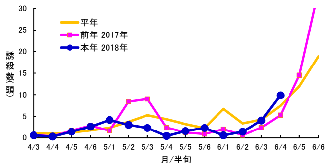
図3 オオタバコガフェロモントラップ誘殺数推移 ※阿波市、三好市、東みよし町、石井町の7地点平均
