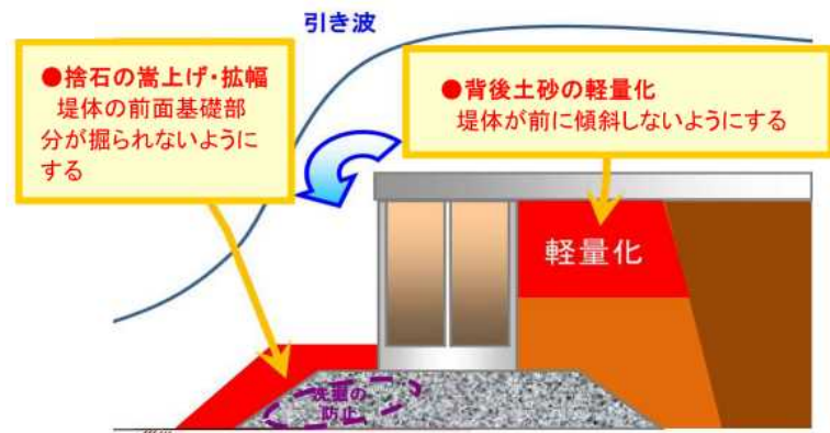
【岸壁の粘り強い化】
