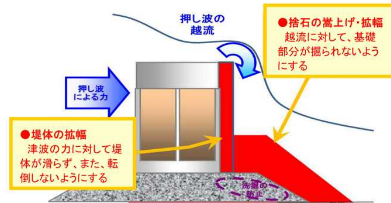
【防波堤の粘り強い化】
