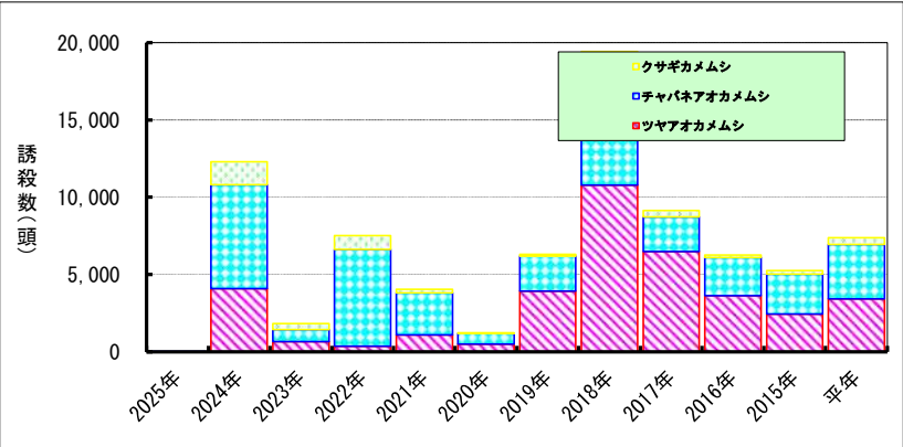
図5 果予察圃場の予察灯への誘殺数(4/1-11/30)
