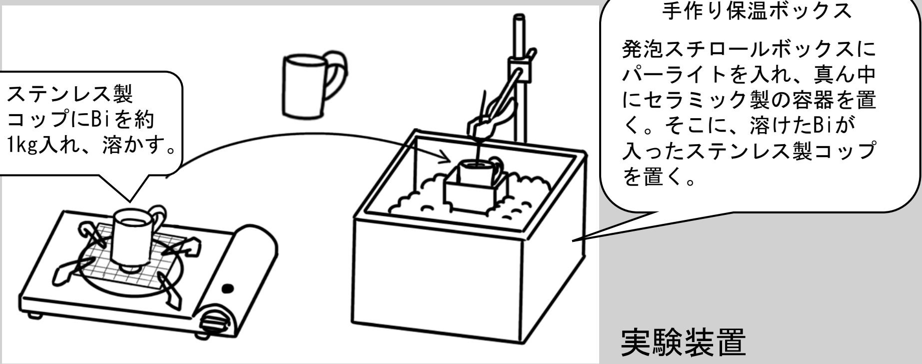
実験装置
