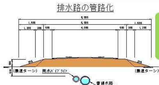
排水路を管路化
