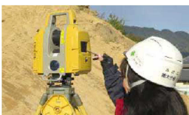
3次元設計データによる作業土工（床掘）を進めるMGバックホウとワンマン3次元測量
