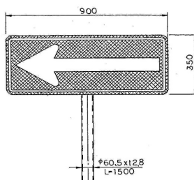
誘導標2型
