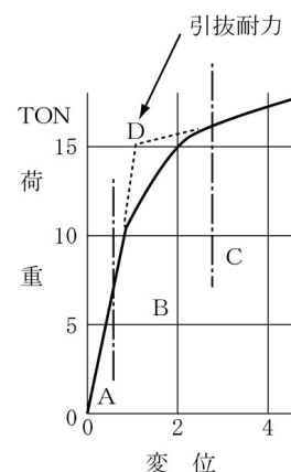
図４－１ ロックボルト引抜試験
