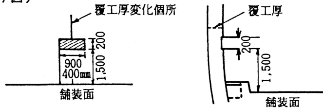
(取付け図)
