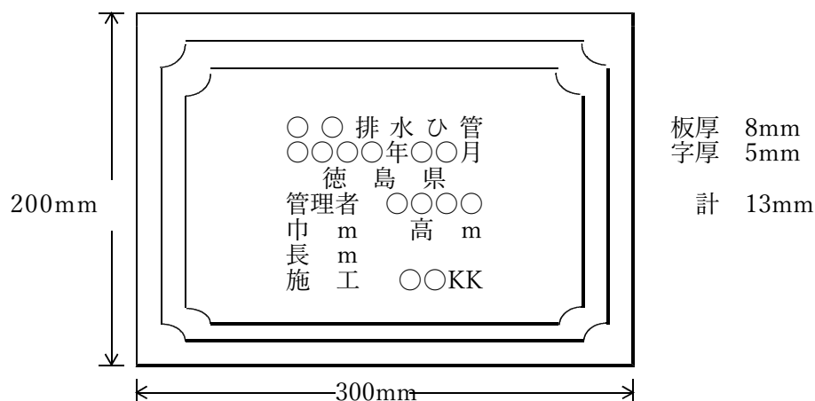
図6-3-1 銘板の寸法及び記載事項
