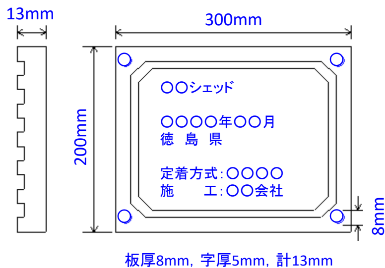
図10-7-1 銘板の寸法及び記載事項
