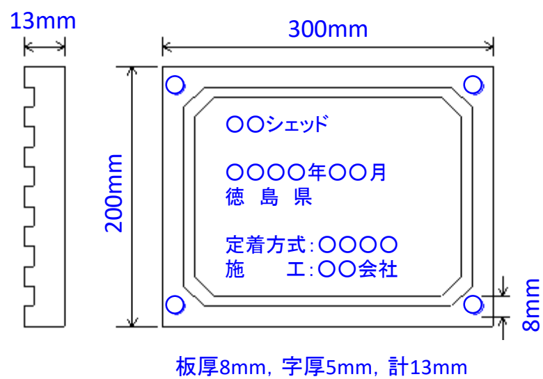
図10-8-1 銘板の寸法及び記載事項
