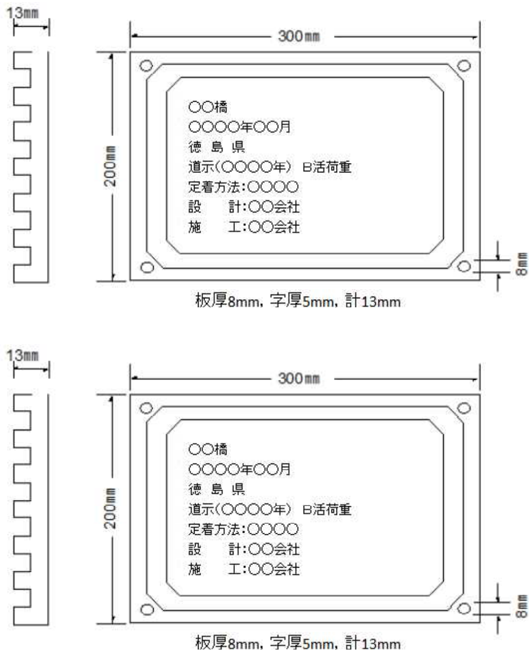
図3-1-2 銘板の寸法及び記載事項
