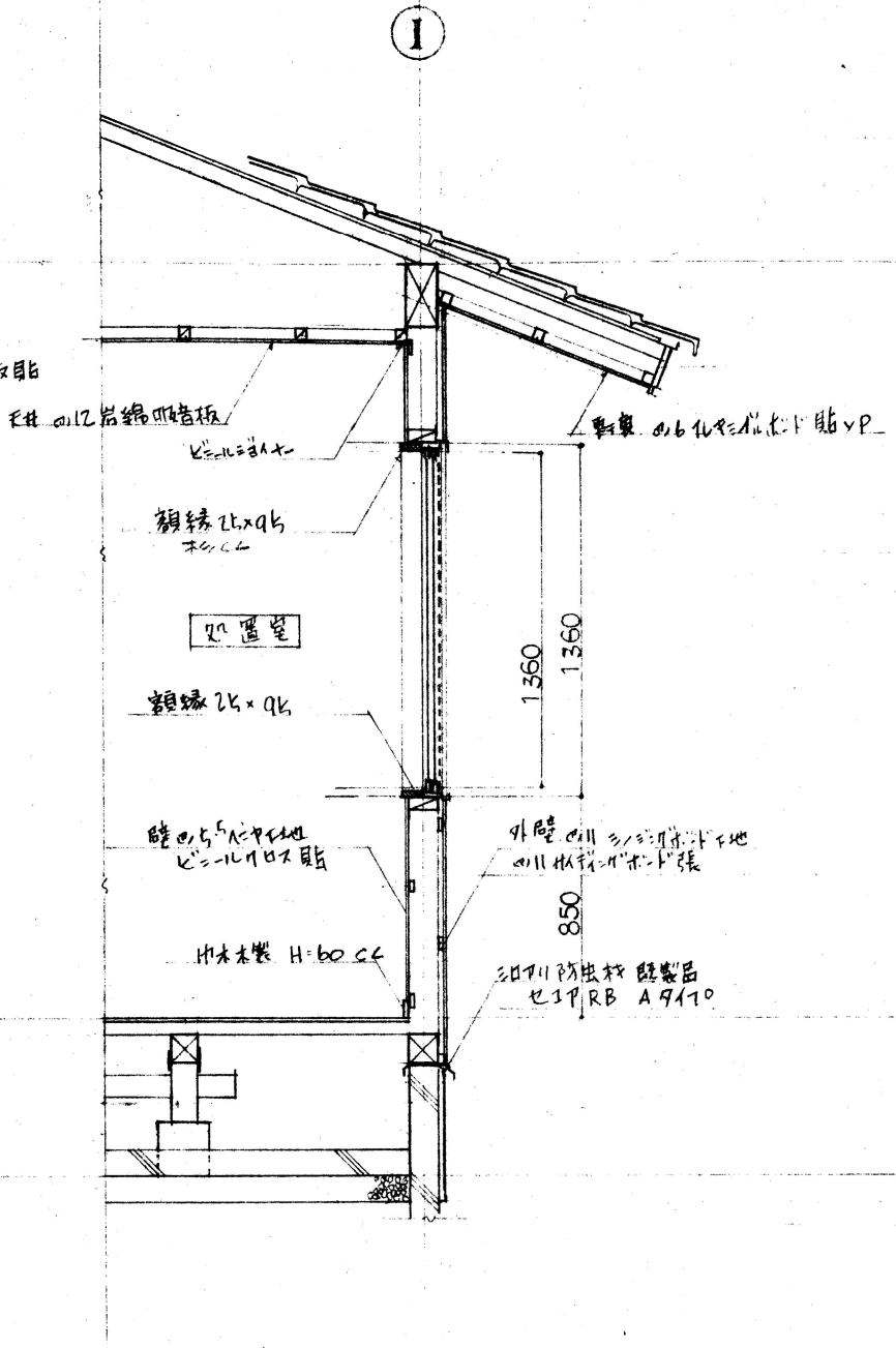
処置室 断面詳細図 S = 1:30
