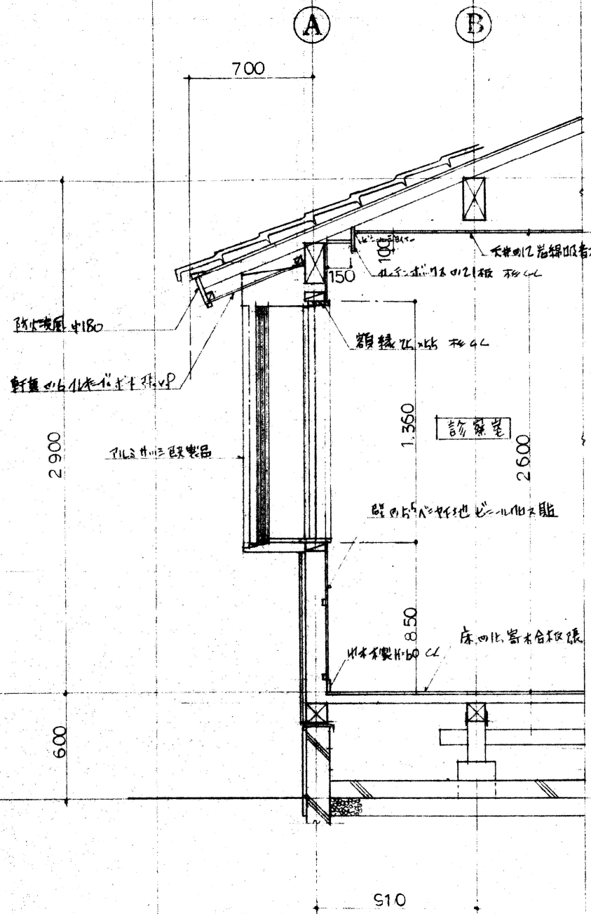
診察室 断面詳細図 S = 1:30
