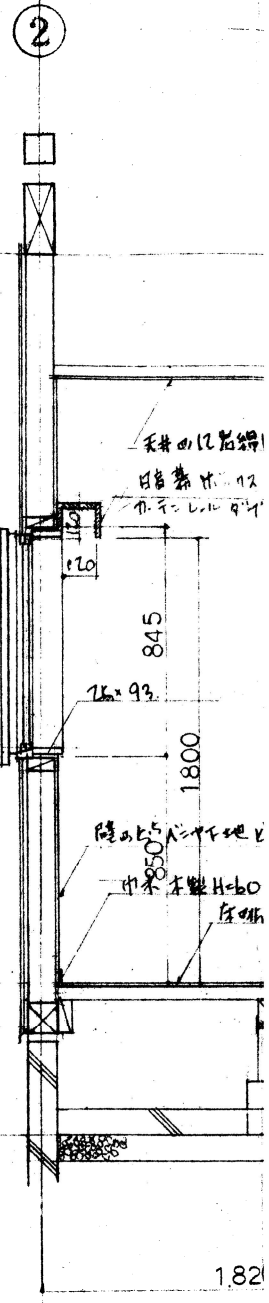
操作室 断面
