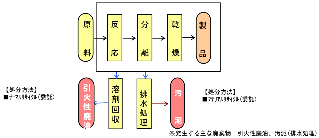
図1 主要な製造工程A [有機化学製品A]
