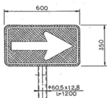
誘導標1型
