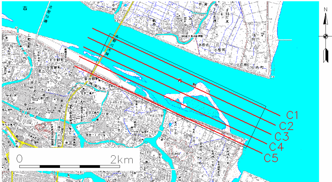
図 3-1-2-1 レザ-測量計測コース図
