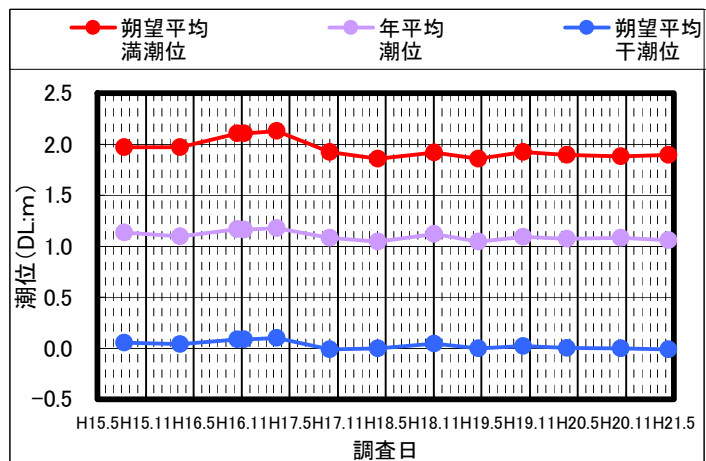
図 3-2-3-3 調査時の潮位
