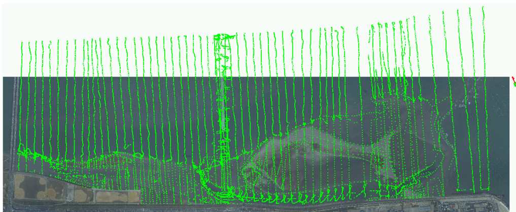
図 3-1-2-2(2) 深浅測量測線（平成 21 年 4 月 3 日～5 日計測）
