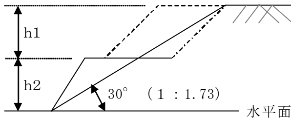
(図4-2) 上下に分離された崖がある場合
