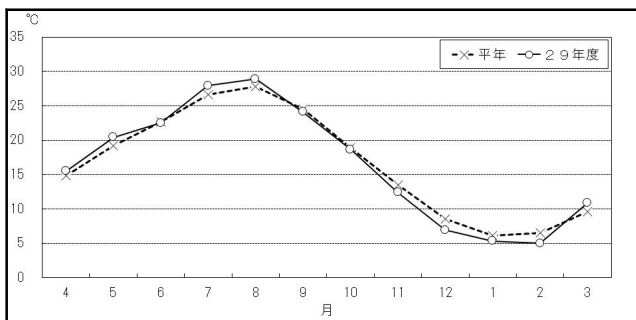
図VI-3 気温の状況
