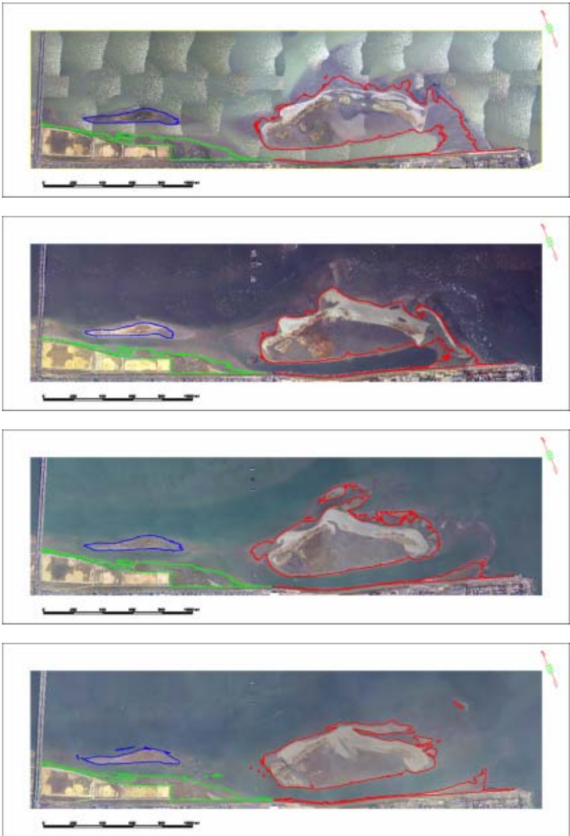
図 1-5-5 港湾D.L.+0.783mでの汀線の変化(上から順にH15年8月11日、H16年3月10日、H16年10月14日、H16年11月8日、背景は各計測時のオルソ画像)
