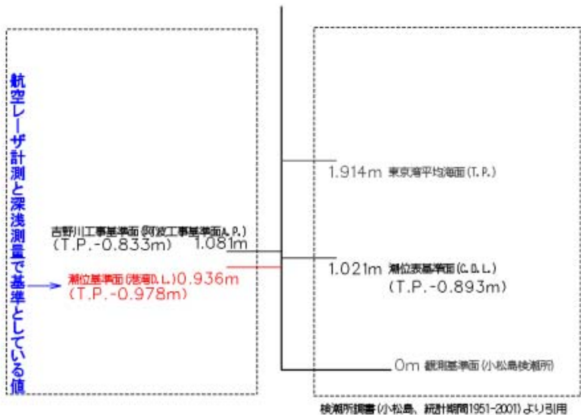
図 1-4-2 潮位及び各種基準面高さの関係
