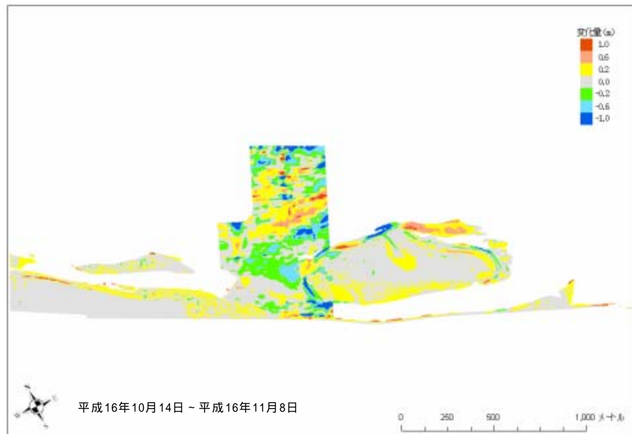
图 1-5-4 地形变化量 (DEM差分)
