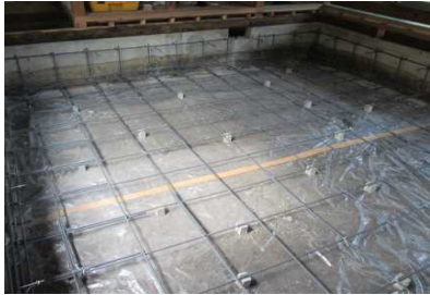
工事中 基礎配筋施工
