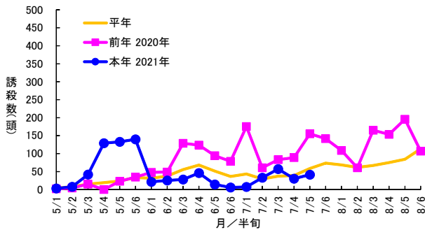
図1 ハスモンヨトウフェロモントラップ誘殺数推移(甘藷圃場)
