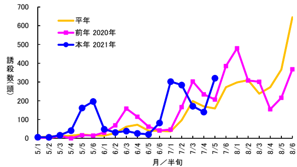
図2 シロイチモジヨトウフェロモントラップ誘殺数推移(甘藷圃場)
