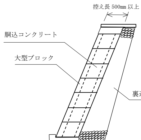
断面図
