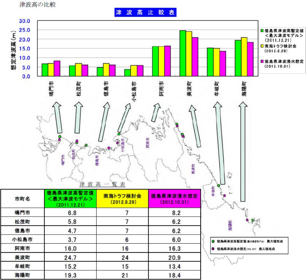
【南海トラフ地震における想定津波高及び津波影響開始時間】
