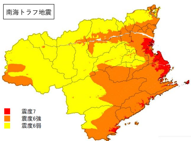
【震度分布】
