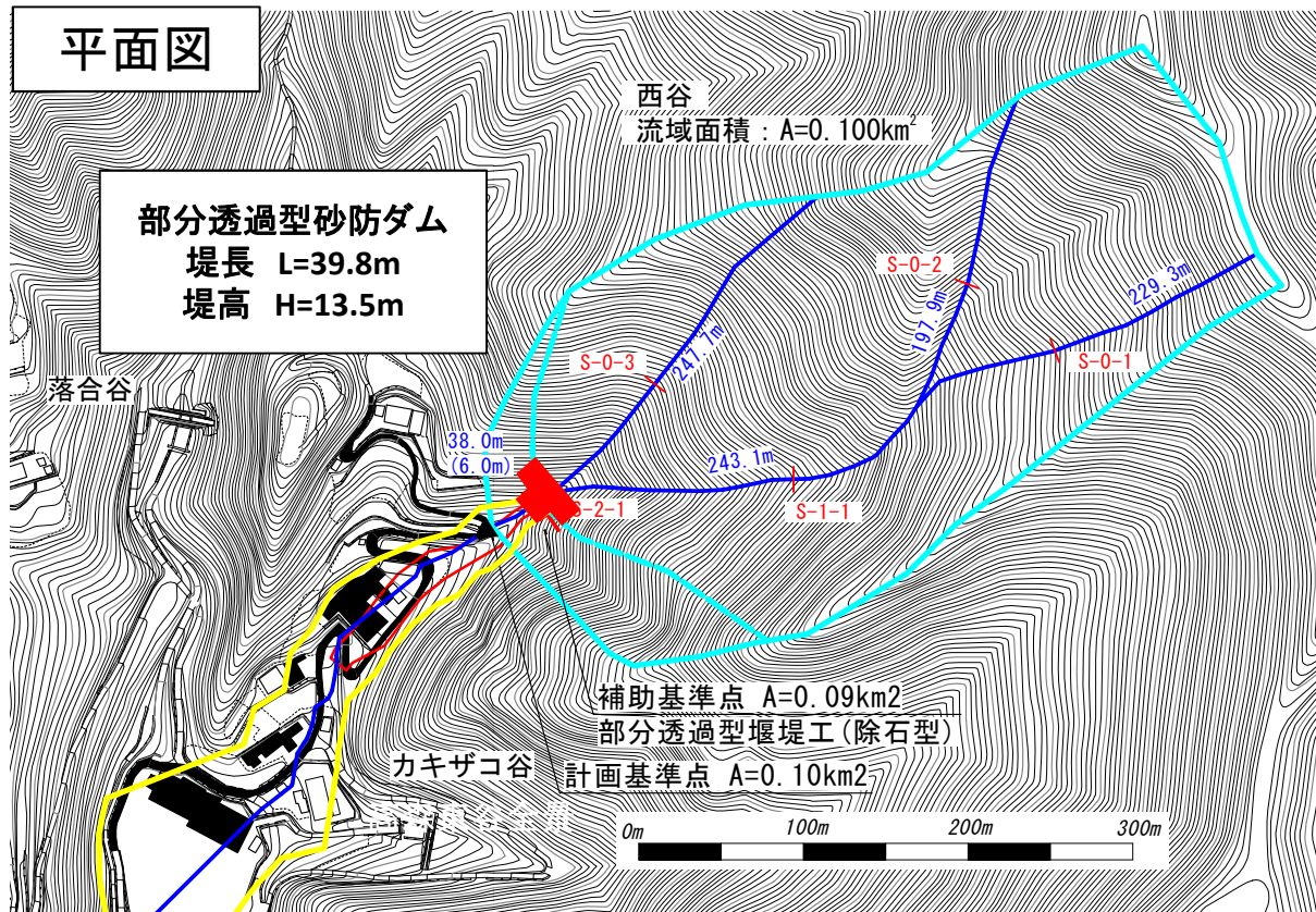
一般図(概略図)
