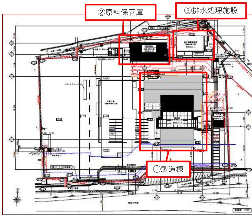
○配置図
