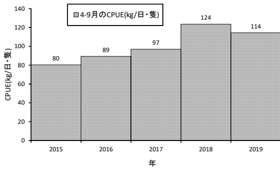
図4. A漁協の小型底びき網による主漁期CPUE (kg/日・隻)の経年変化
