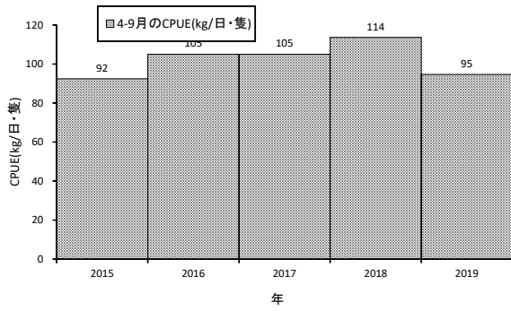
図3. A漁協の延縄による主漁期CPUE (kg/日・隻)の経年変化
