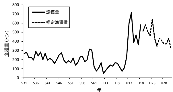
図2. 漁獲量の経年変化
