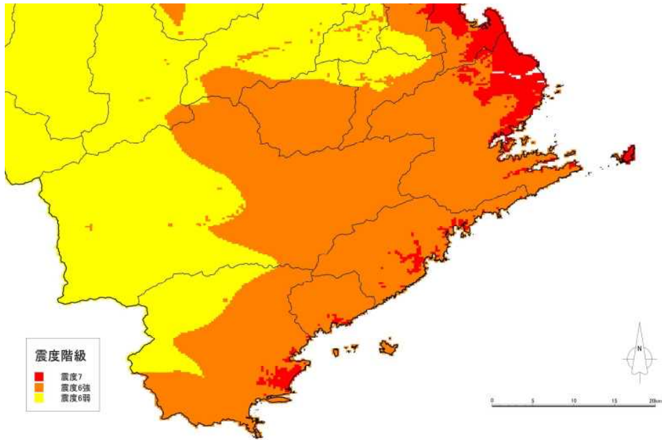
【資料】南海トラフ巨大地震による震度分布
