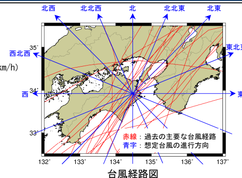
台風経路図
