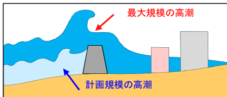
対象とする高潮のイメージ
