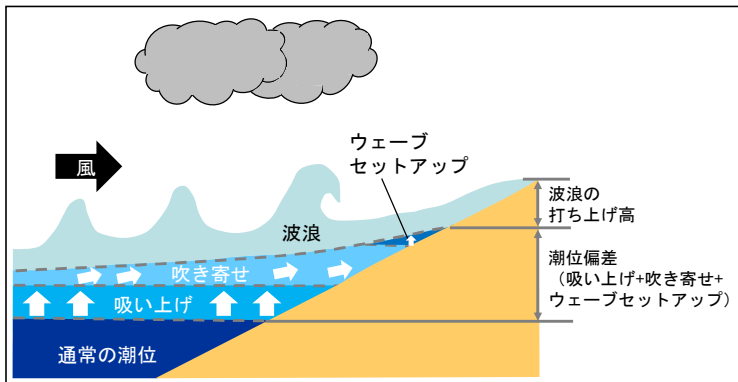
高潮の発生メカニズム
