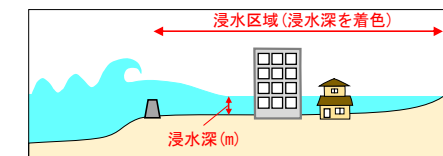
浸水区域と浸水深の定義
