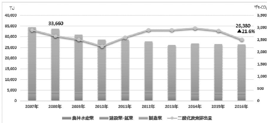
産業部門における業種別エネルギー消費量及び二酸化炭素排出量の推移
