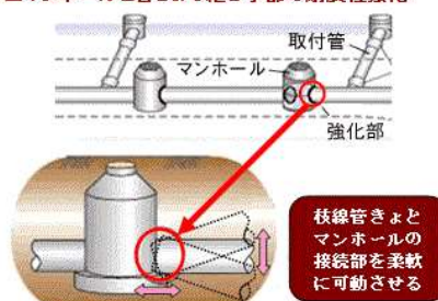
■マンホールと管ぎょの継ぎ手部の耐震性強化
