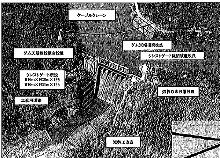
長安口ダム改造事業全体図
