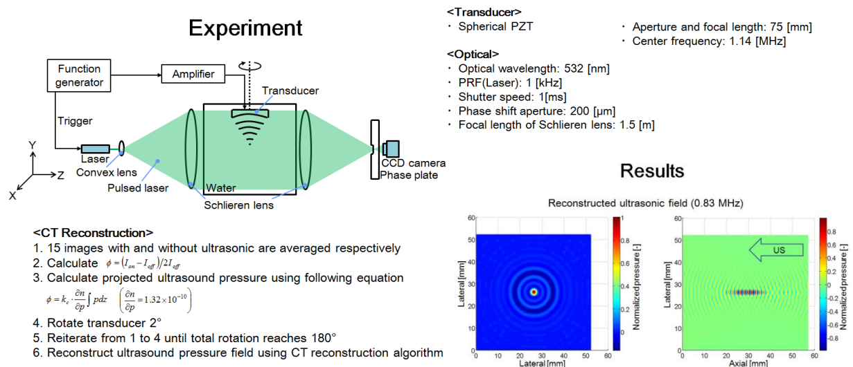
図 8 位相コントラスト法の測定系
