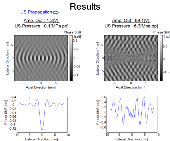
図 10 高音圧における位相ラップ
