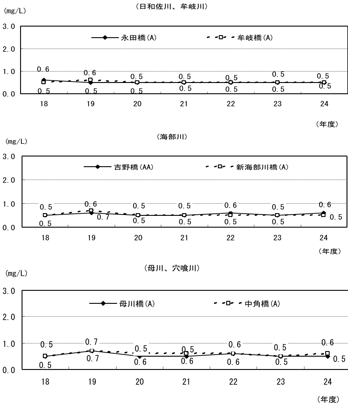
図2-2-19 BOD平均値の経年変化（県南沿岸海域に流入する河川）
