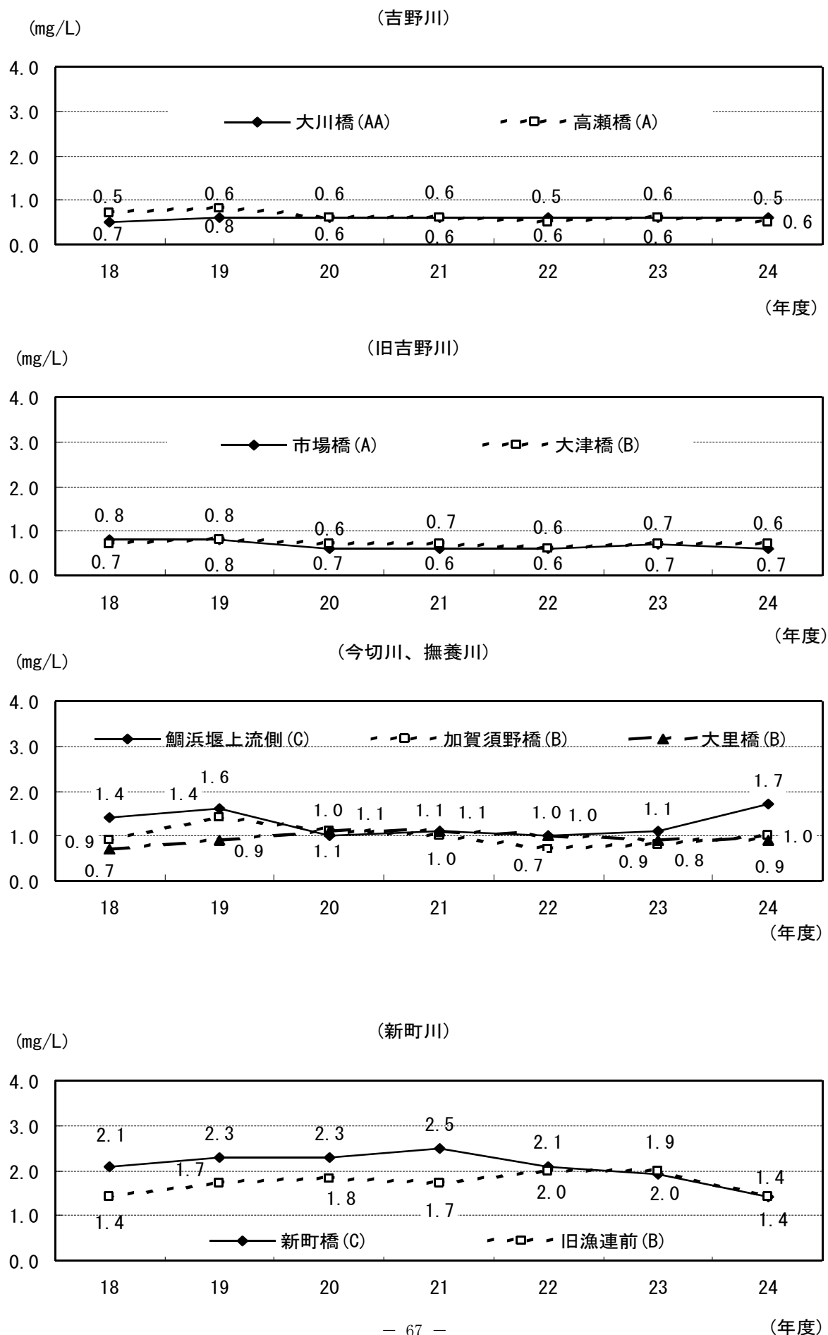
図2-2-13 BOD平均値の経年変化（吉野川水系）
