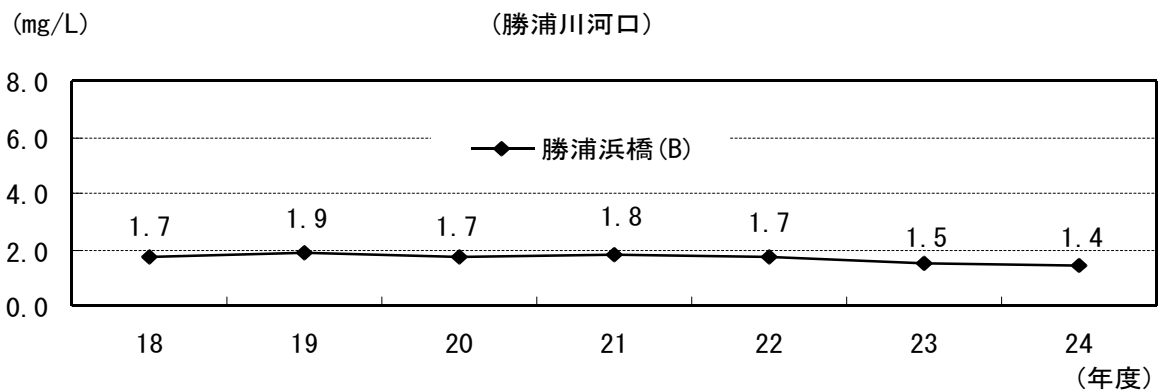
図2-2-27 COD平均値の経年変化（港湾等）
