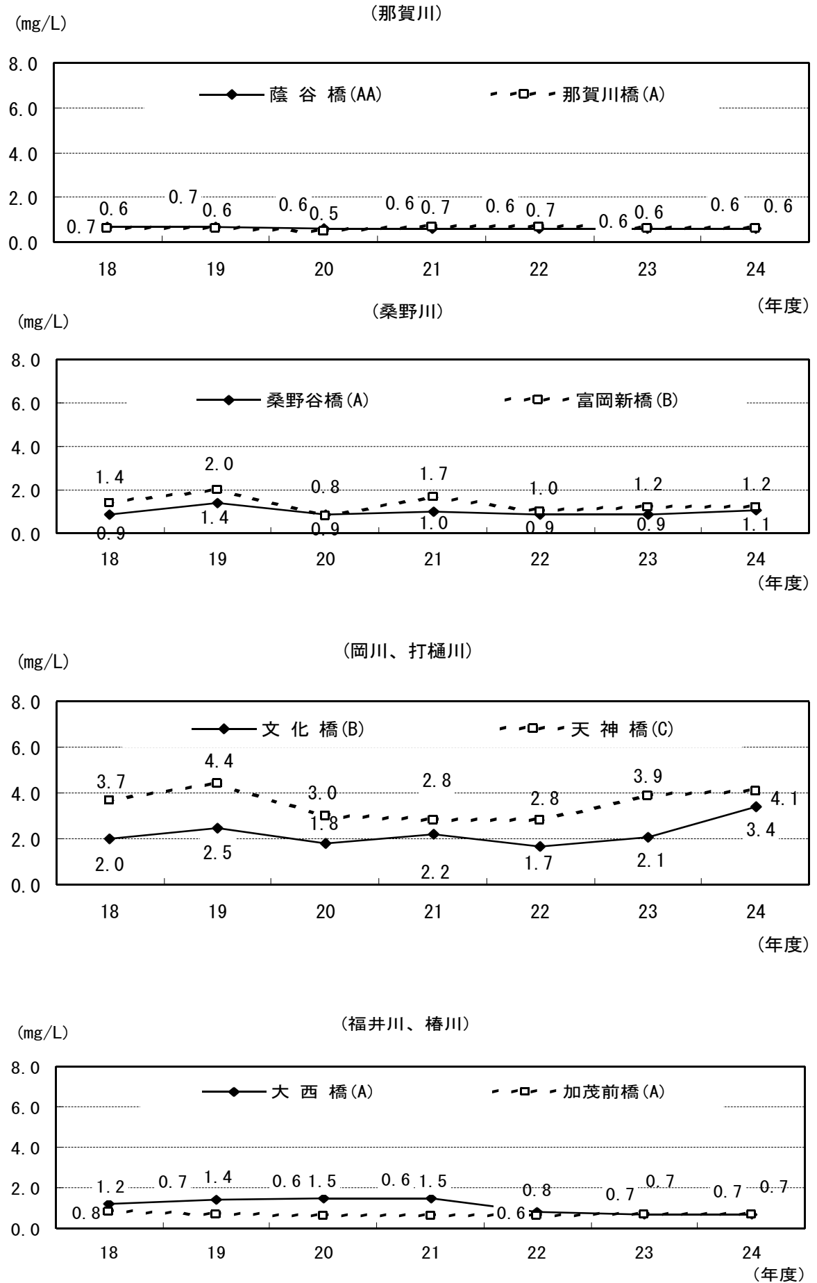
図2-2-17 BOD平均値の経年変化（那賀川水系等）
