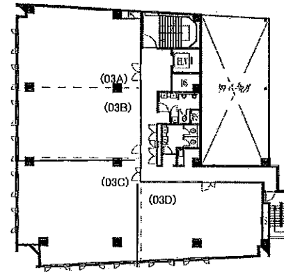
3階平面図
