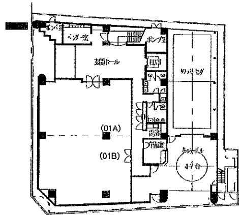
1階平面図
