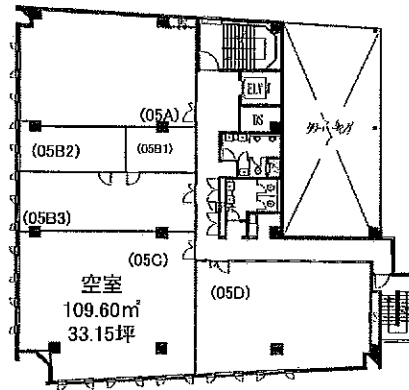
5階平面図
