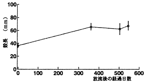
図5 牟岐町ねりぐろみにおけるメガイ人工種苗の放流後の成長 放流は1991年8月9日 標準偏差を垂直線で示す
