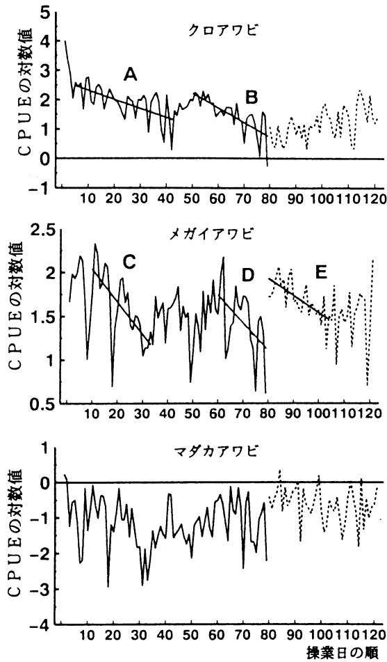
図1 1992年牟岐町地先におけるクロアワビ（上段）、メガイアワビ（中段）およびマダカアワビの単位努力量当たり漁獲個体数（CPUE）の日変化 （CPUE：個体数／人・2.5時間）A～Eは本文参照
