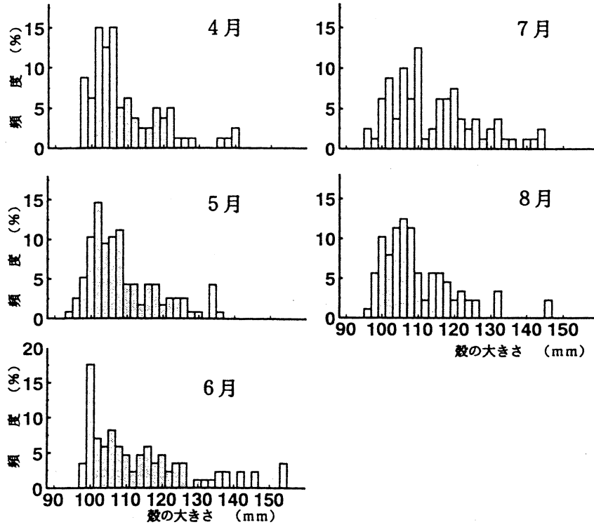
図3 牟岐町地先におけるメガイアワビの殻長組成の季節変化 (1992年調査資料)
