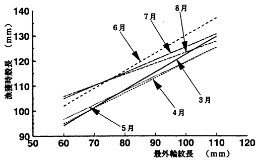
図10 牟岐町地先のマダカアワビの最外輪紋長と漁獲時殻長の月別変化
