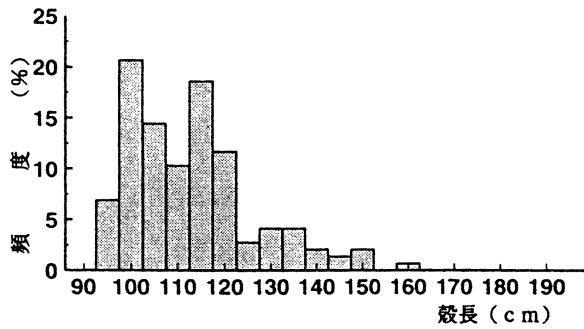
図4 牟岐町地先におけるメダカアワビの殻長組成 1992年4月～8月測定
