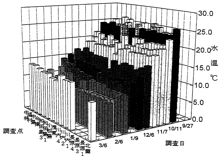
図2 水温鳥瞰図
