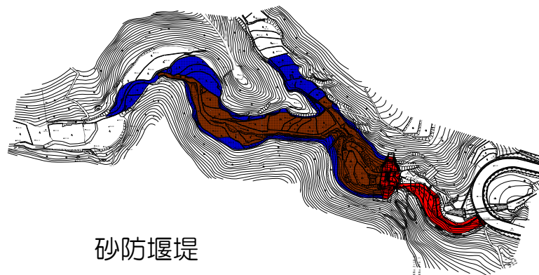
砂防堰堤位置
