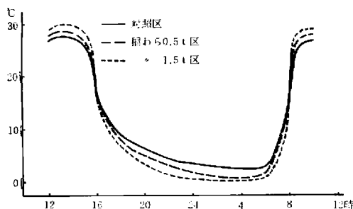
第2図 ハウス内温度の日周変化(2月2日~3日) 稲わらの施用量と温度の変化
