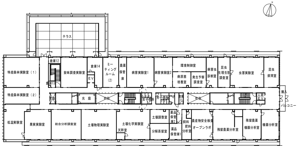
3階 平面図
