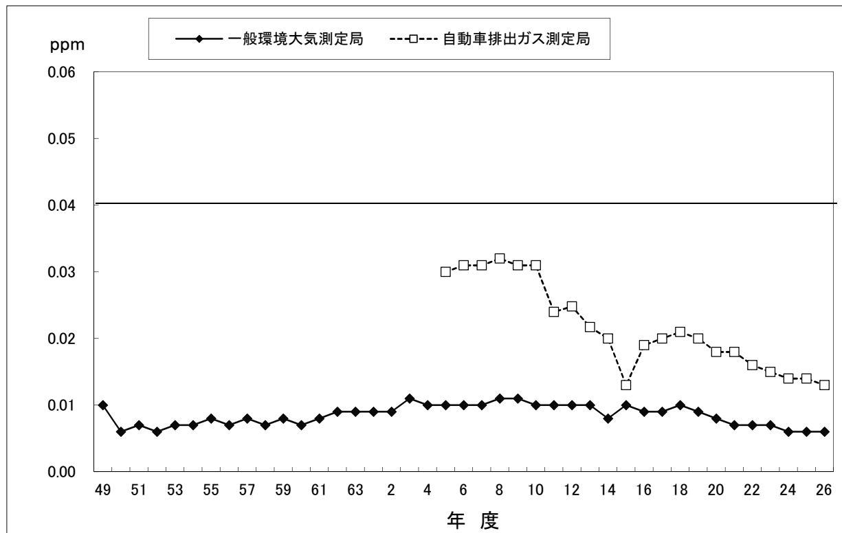
二酸化窒素年平均値の経年変化 (一般局：有効測定局平均、自排局1局)
