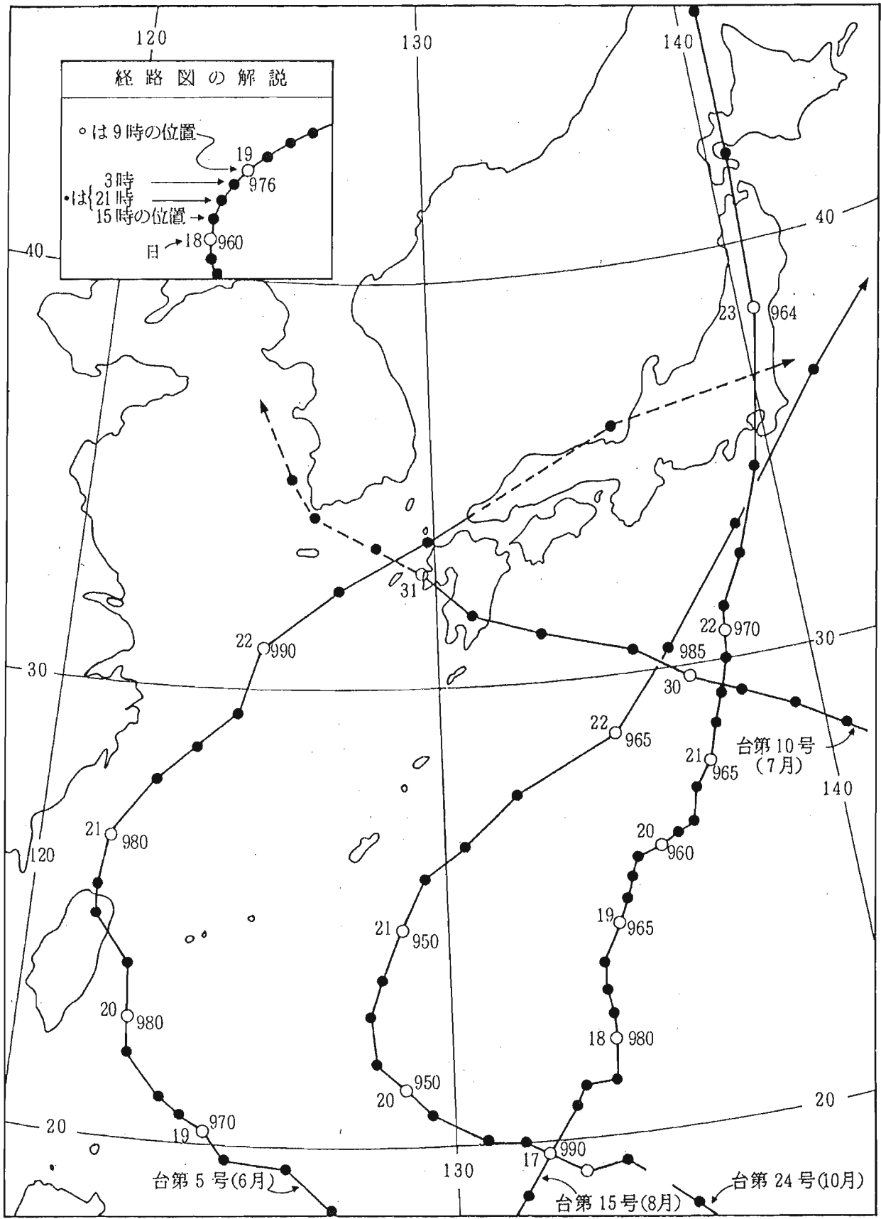
台 風 経 路 図
