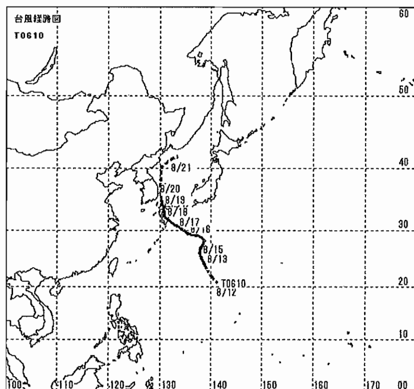
台風第10号経路図（8月17日～19日）
