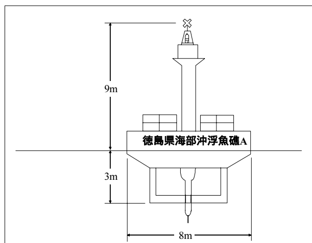
図2 浮魚礁の構造
