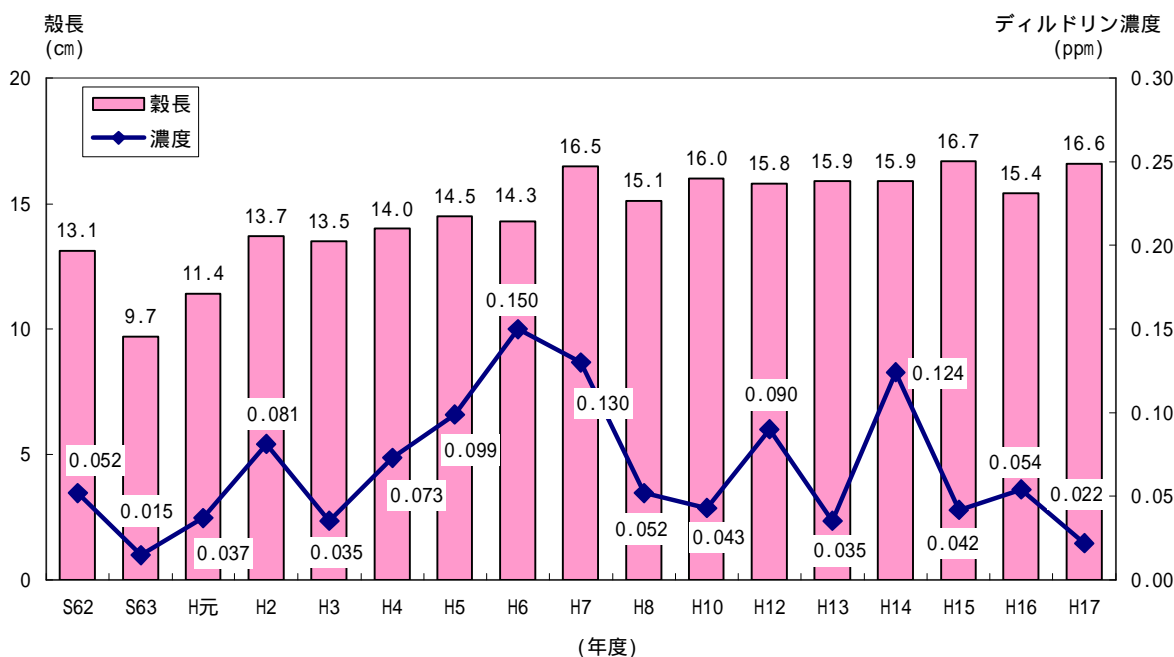
図2-35 イガイ中のディルドリン濃度（平均値）
